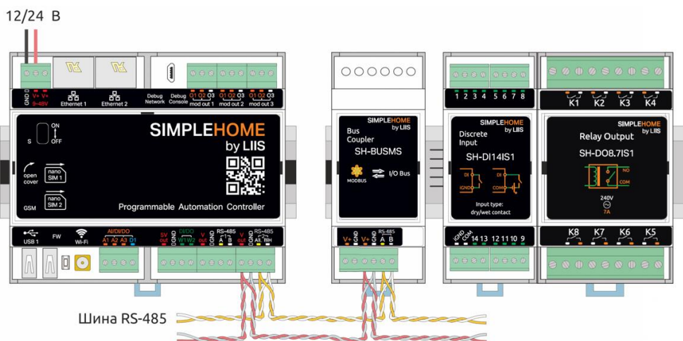
Примеры соединений SH-BUSMS
