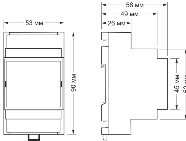
Габаритные размеры SH-CHOI3.10MS1
