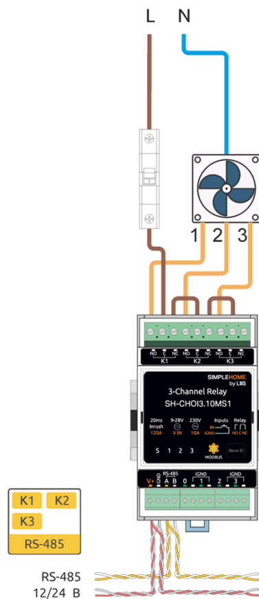
Пример схемы подключения SH-CHOI3.10MS1
